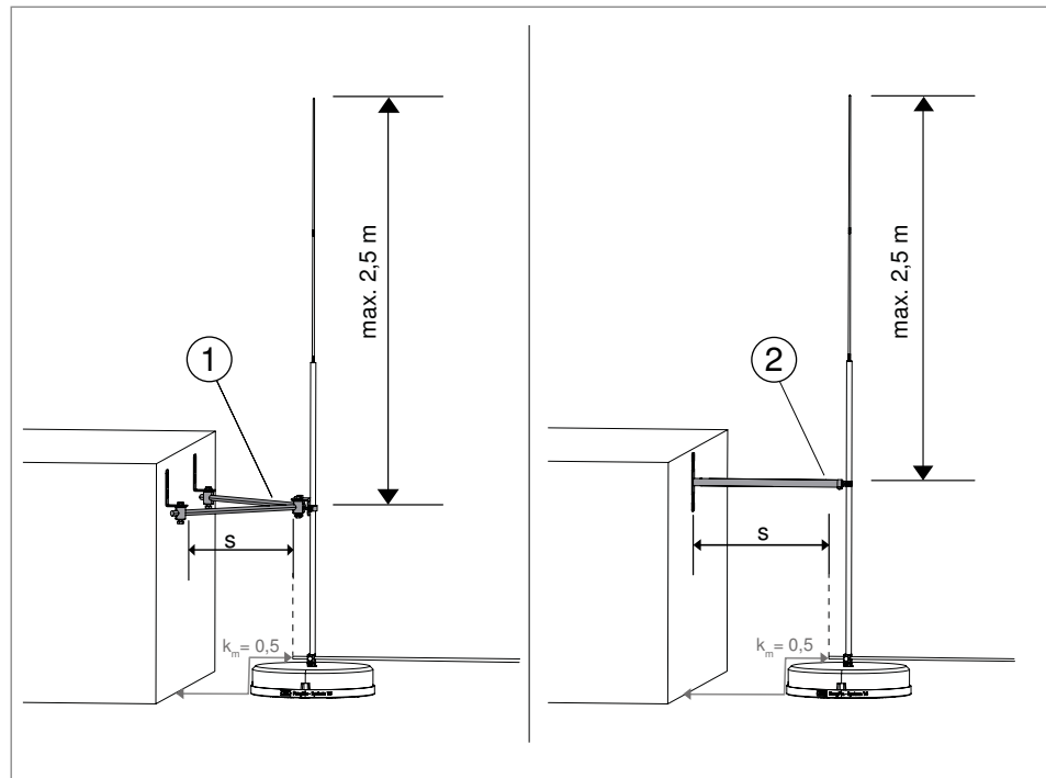
Abb. 2: Mechanische Befestigung der Fangstange
