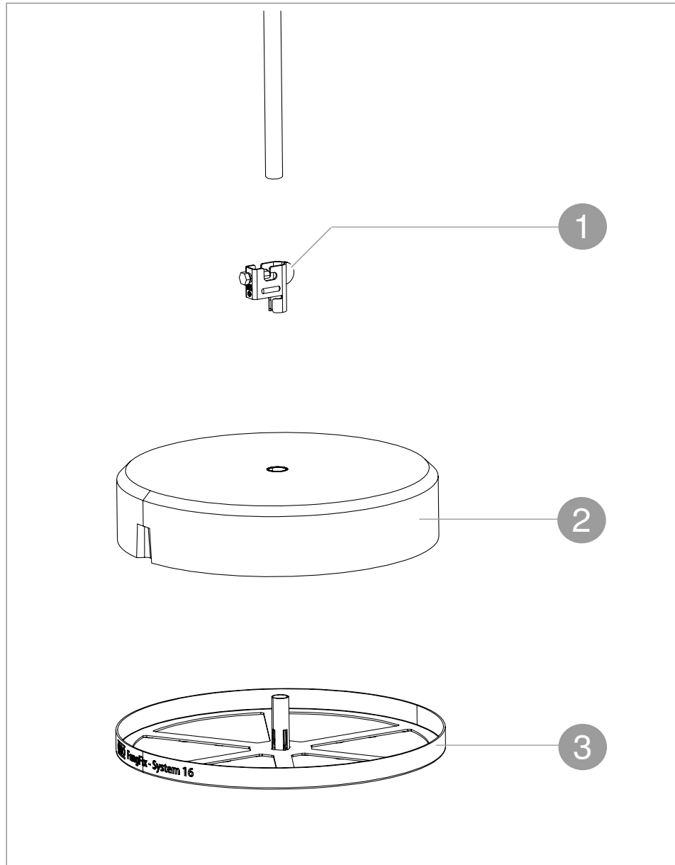
Abb. 1: Systemübersicht
