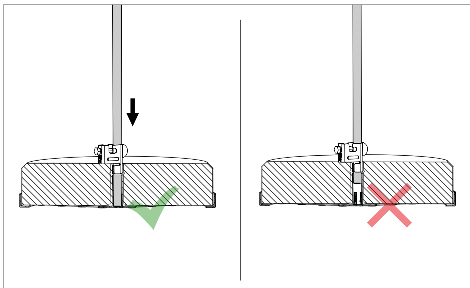
Abb. 5: Fangstange montieren
