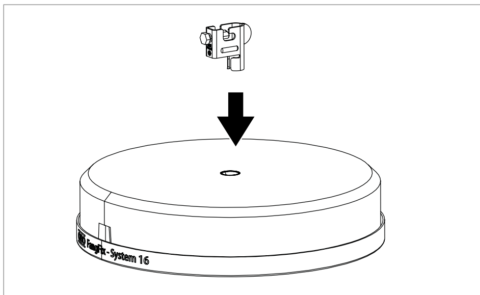
Abb. 4: FangFix-Klemme montieren
