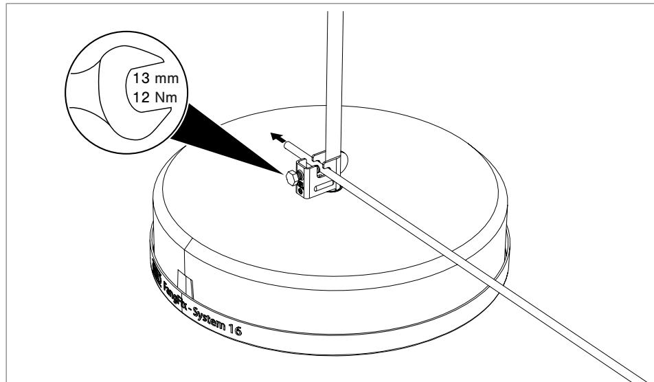
Abb. 6: Rundleiter anschließen
