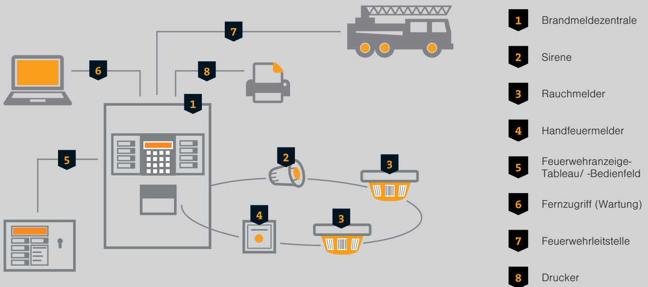
Schematischer Aufbau einer modernen Brandmeldeanlage
