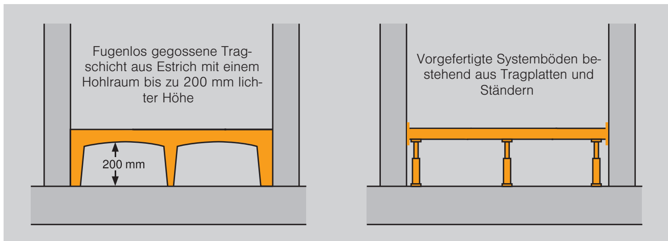
Definition von Systemböden: Hohlboden (links), Doppelboden (rechts)
