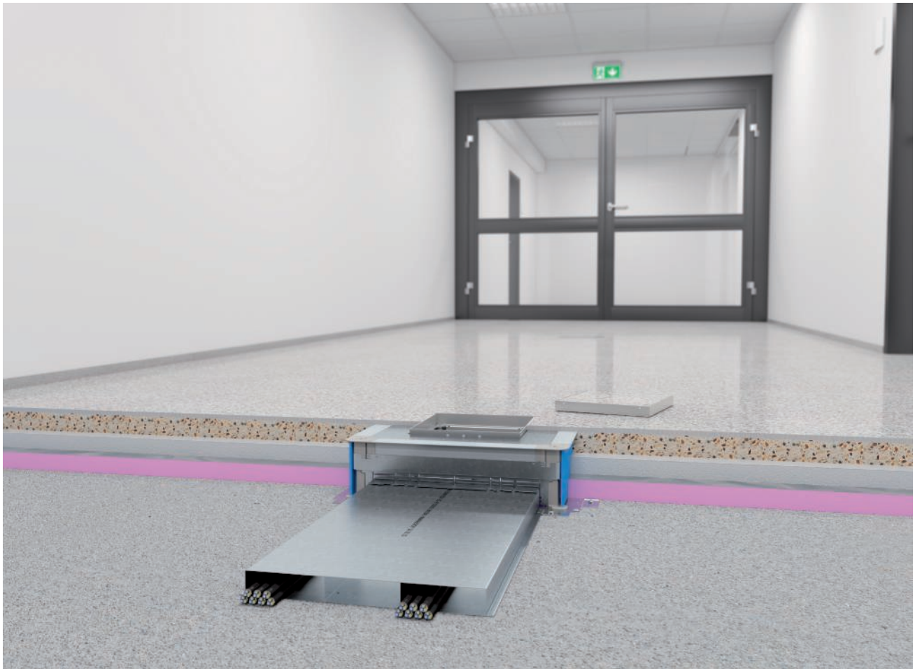
Estrichüberdecktes Kanalsystem EÜK
