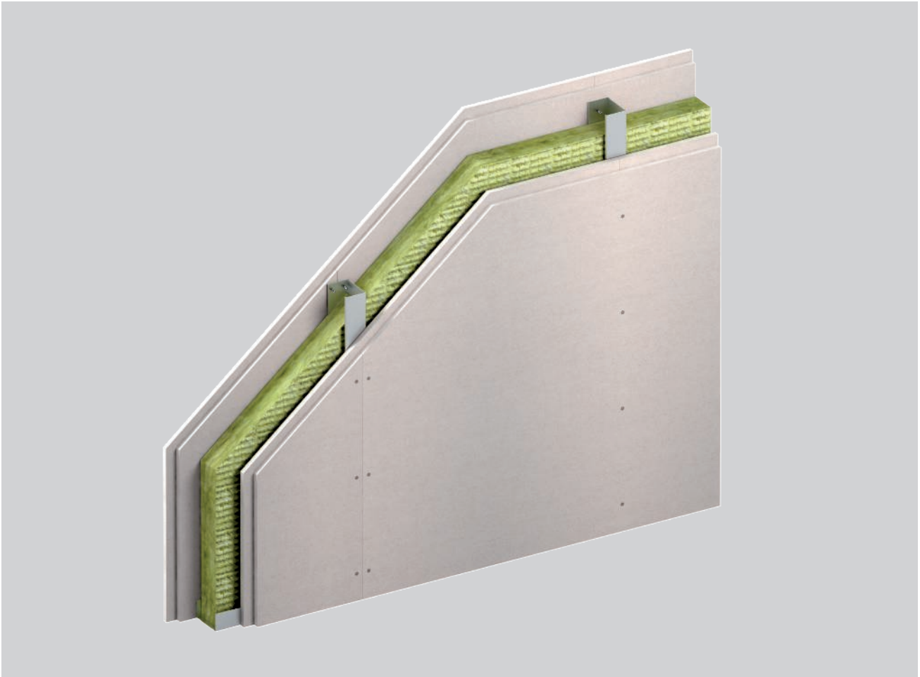
Trennwandkonstruktion mit Gipskartonplatten
