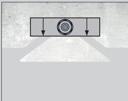
Betonkantenbruch
