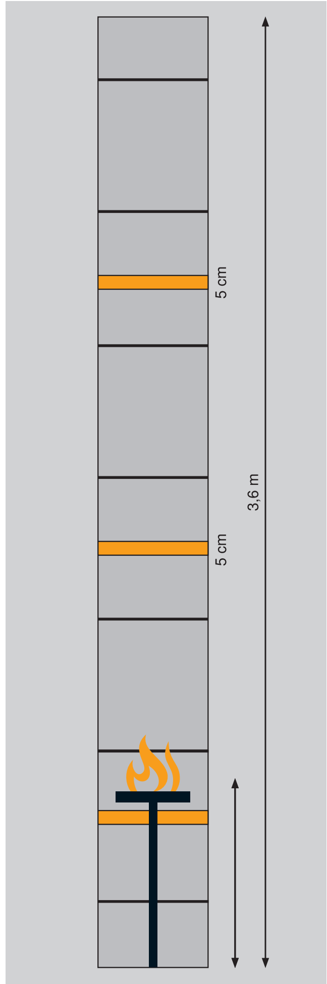
Aufbauprinzip IEC-Prüfung
