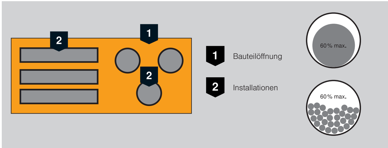
Maximal 60 % der Fläche darf mit Kabeln, Tragsystemen, Rohren usw. belegt werden
