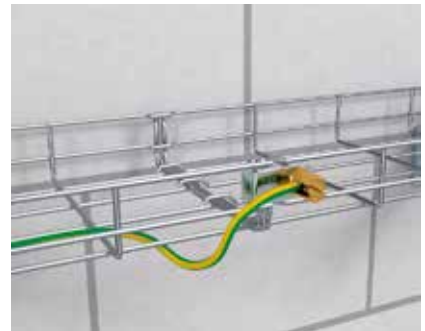
Erdungsklemme/Erdanschluß Erdungsklemme zur Befestigung des Potentialausgleichleiters am Kabeltragsystem.
